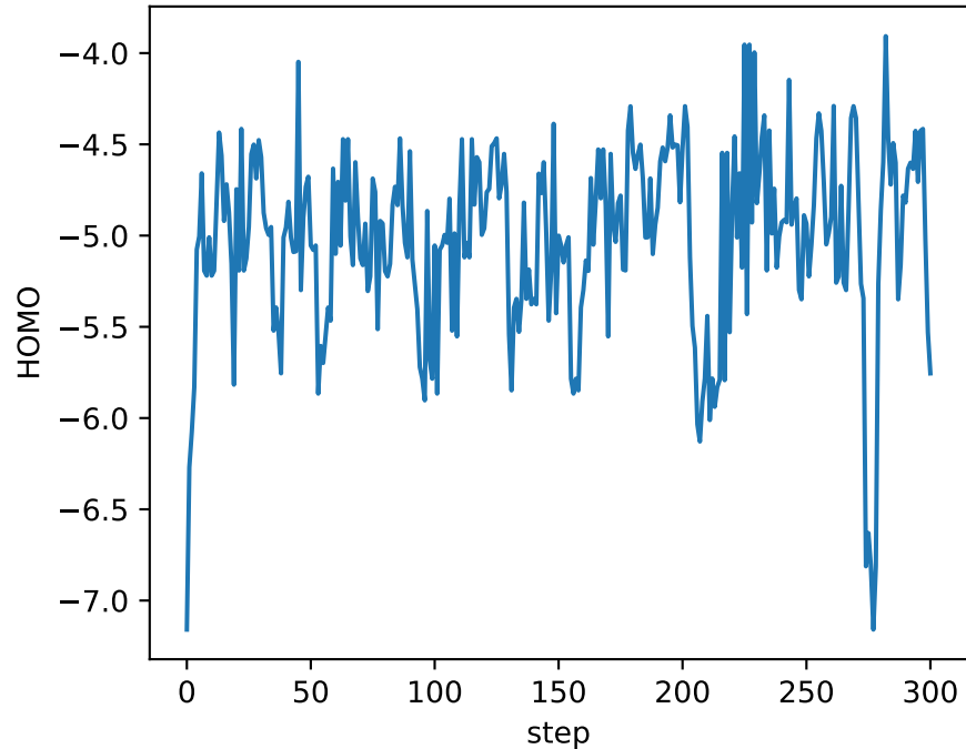
HOMO - evolution
